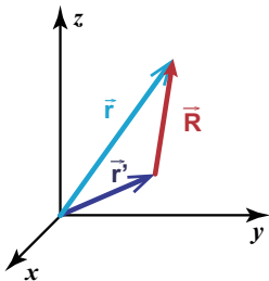
Figure 1: 直角坐标系中的位置矢量。
