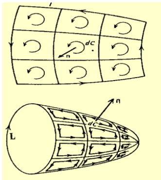
Figure 11: 斯托克斯定理
