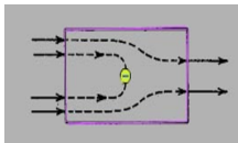
Figure 7: 矢量场通量的性质
