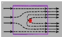
Figure 6: 矢量场的通量
