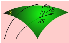
图4 矢量场的通量
