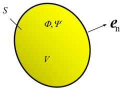
Figure 12: 格林定理示意图
