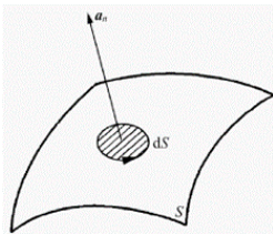
Figure 4: 开曲面上的面元
